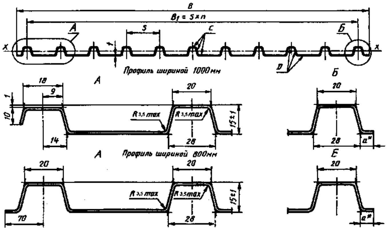
Рисунок 8 - Профилированный лист типа С высотой 15 мм
