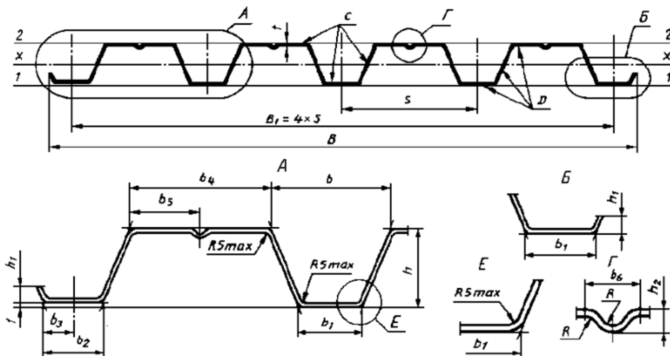
Рисунок 1 - Профилированный лист типа Н высотой 57 и 60 мм
